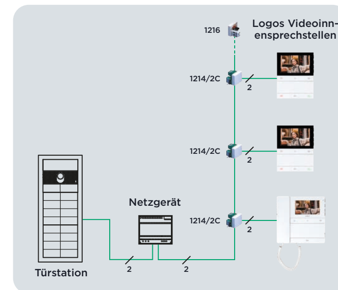
FÜR WOHNKOMPLEXE ODER MEHRFAMILIENHÄUSER
