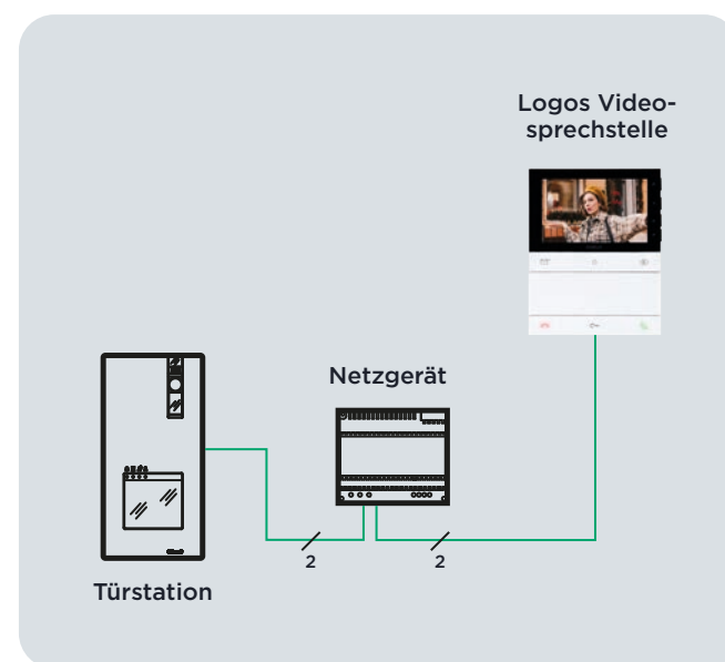
FÜR EIN- BIS VIER-FAMILIENHÄUSER
