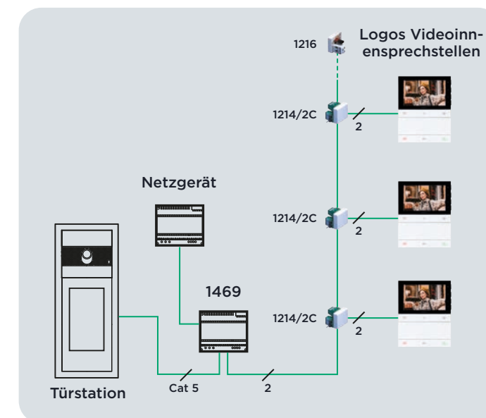
FÜR IP-SYSTEME (erweitert durch ein 1469-Modul)
