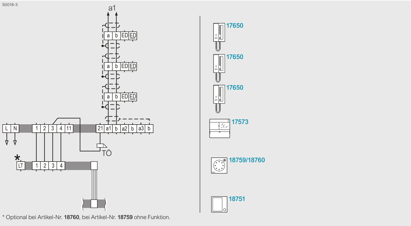
Ein- oder Mehrfamilienhaus mit einer Hauptbuslinie
