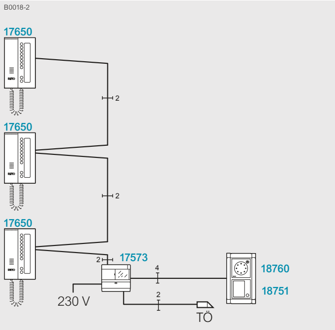
Ein- oder Mehrfamilienhaus mit einer Hauptbuslinie
