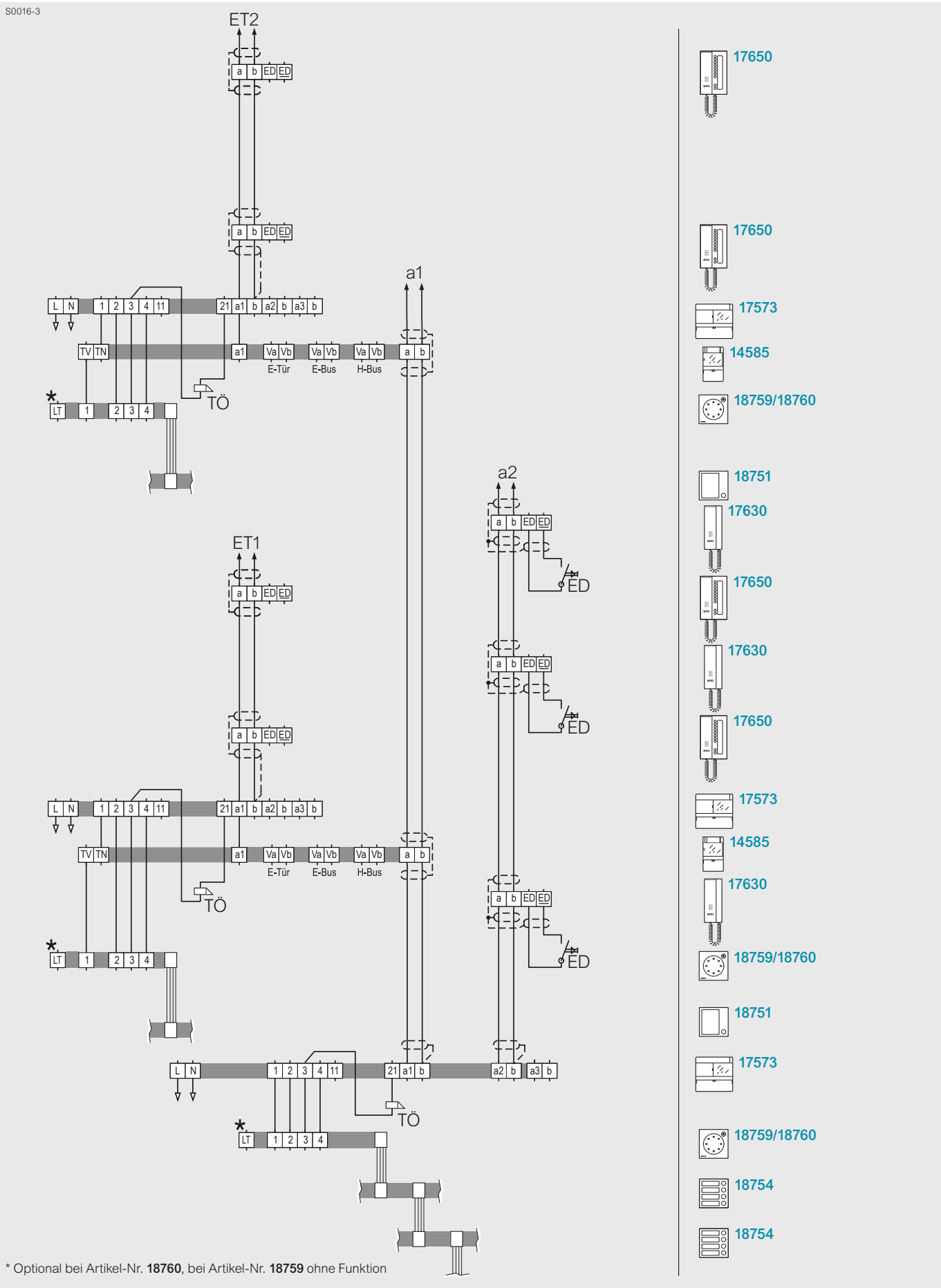
Mehrfamilien- und Geschäftshaus mit separaten Etagentürstationen
