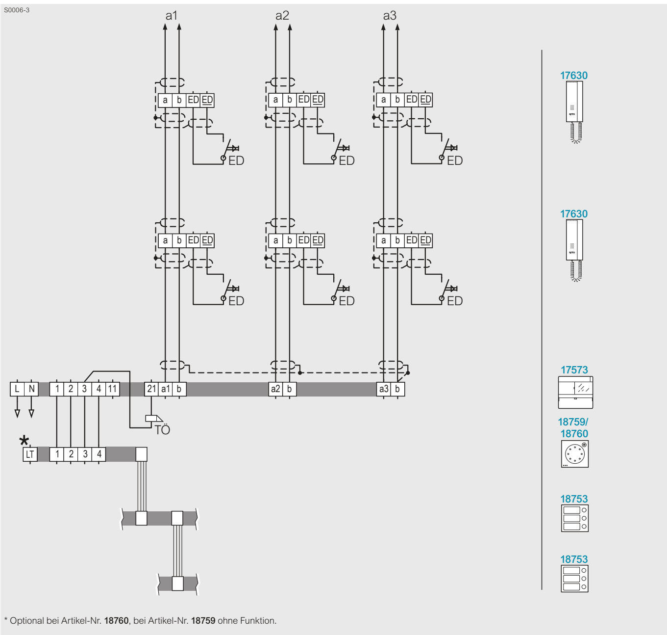
Ein- oder Mehrfamilienhaus mit ein bis drei Hauptbuslinien
