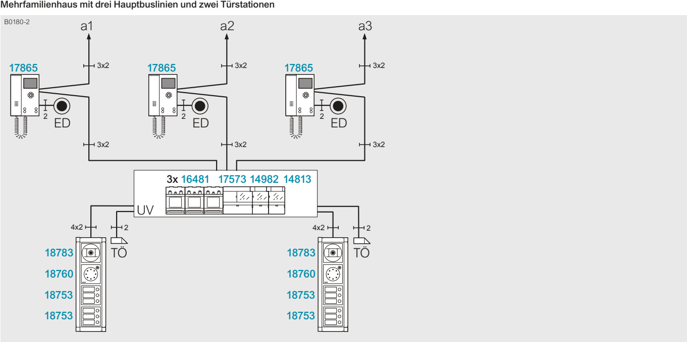
Mehrfamilienhaus mit drei Hauptbuslinien und 2 Türstationen (zentrale Spannungsversorgung)
