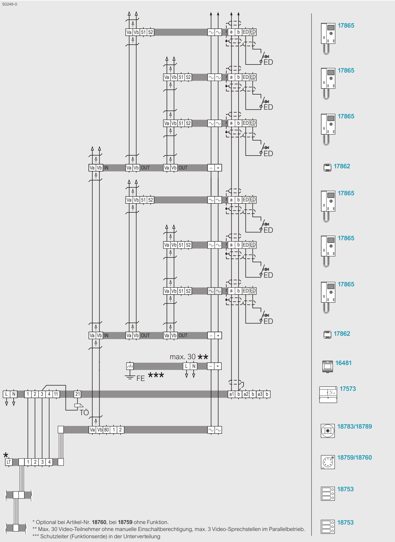
Video-Türsprechanlage im Mehrfamilienhaus mit Steigleitung im Treppenhaus
