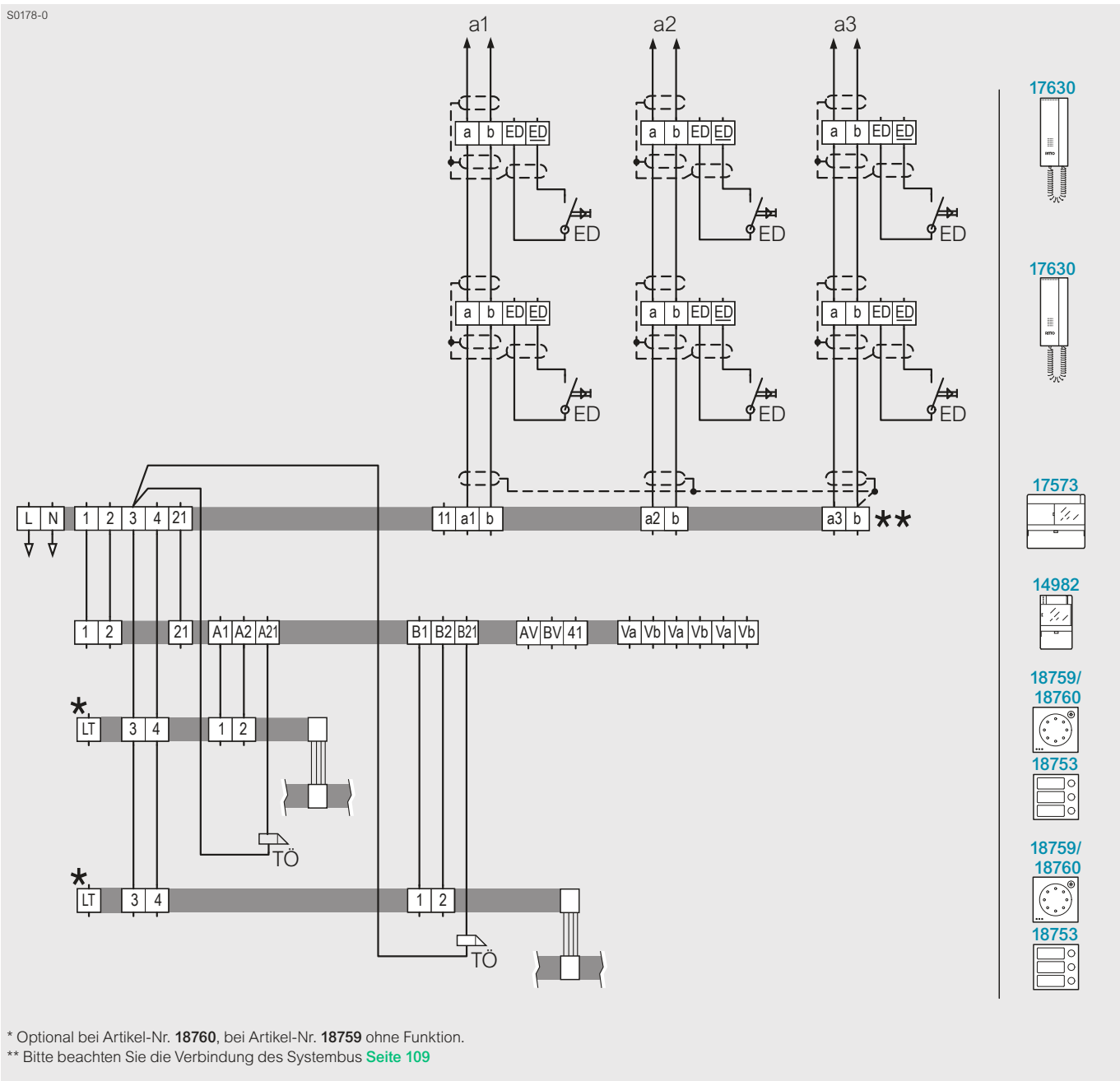
Ein- oder Mehrfamilienhaus mit Erweiterung auf zwei Türstationen
