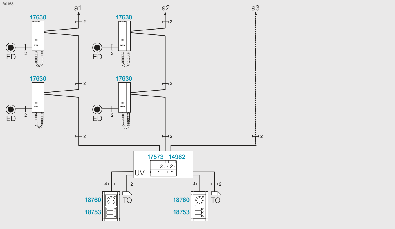
Türumschaltung Artikel-Nr. 14982
