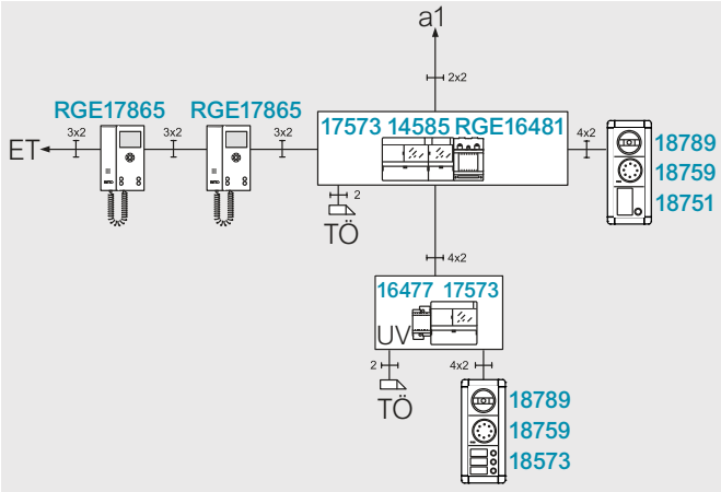
Video-Türsprechanlage für das Mehrfamilienhaus bzw. Geschäftshaus mit separaten Etagenürstationen
