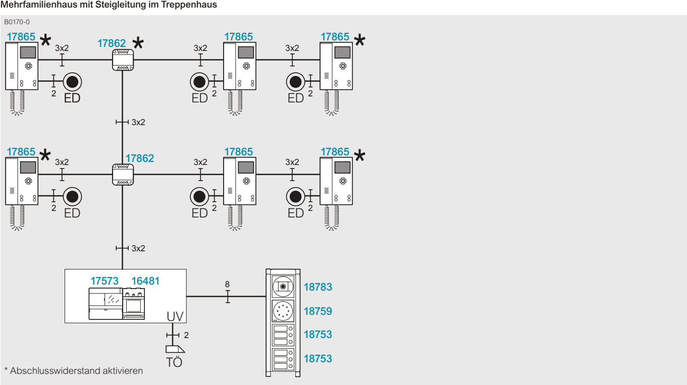
Video-Türsprechanlage im Mehrfamilienhaus mit Steigleitung im Treppenhaus
