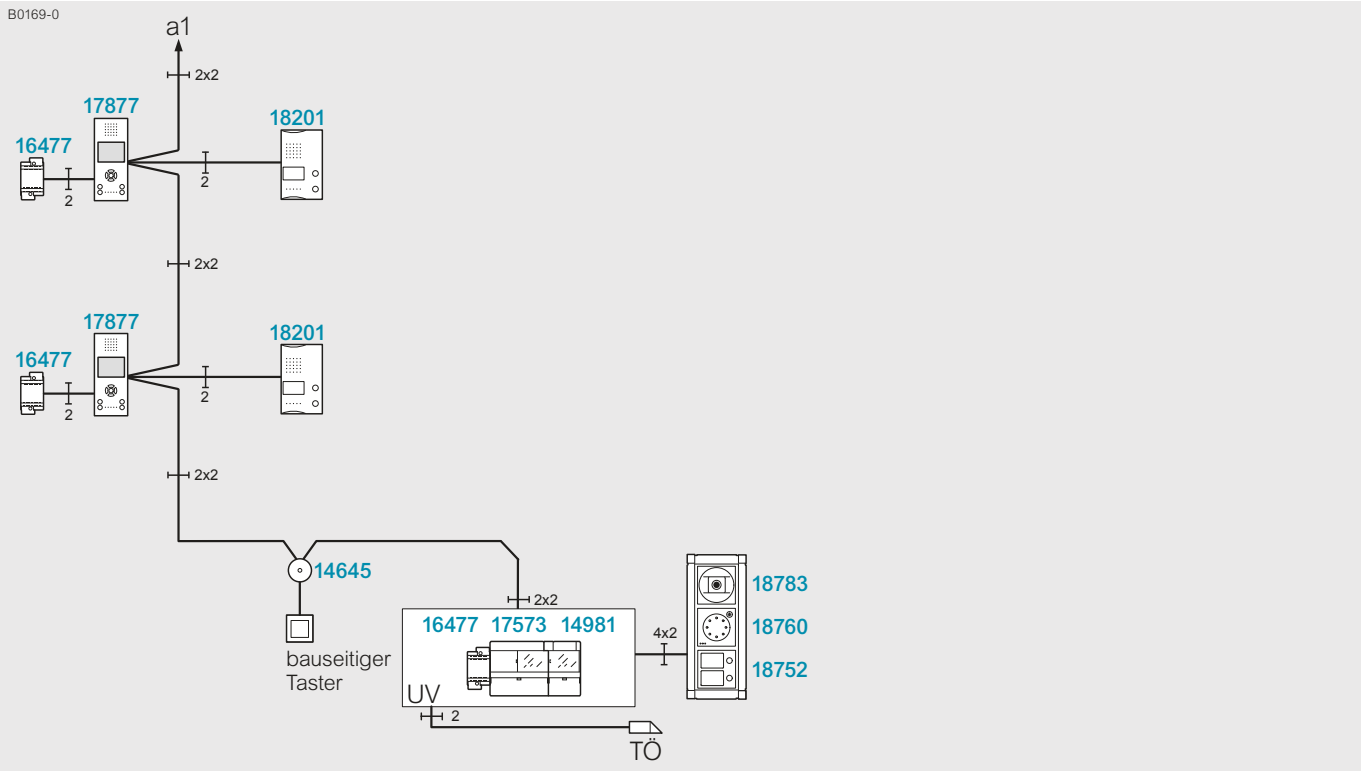
Mehrfamilienhaus mit 2 Teilnehmern und Treppenhaus-Türstation für die Kommunikation zwischen Treppenhaus und Wohnung, sowie Tastenadapter und Schaltgerät z.B. zum einschalten der Treppenhausbeleuchtung
